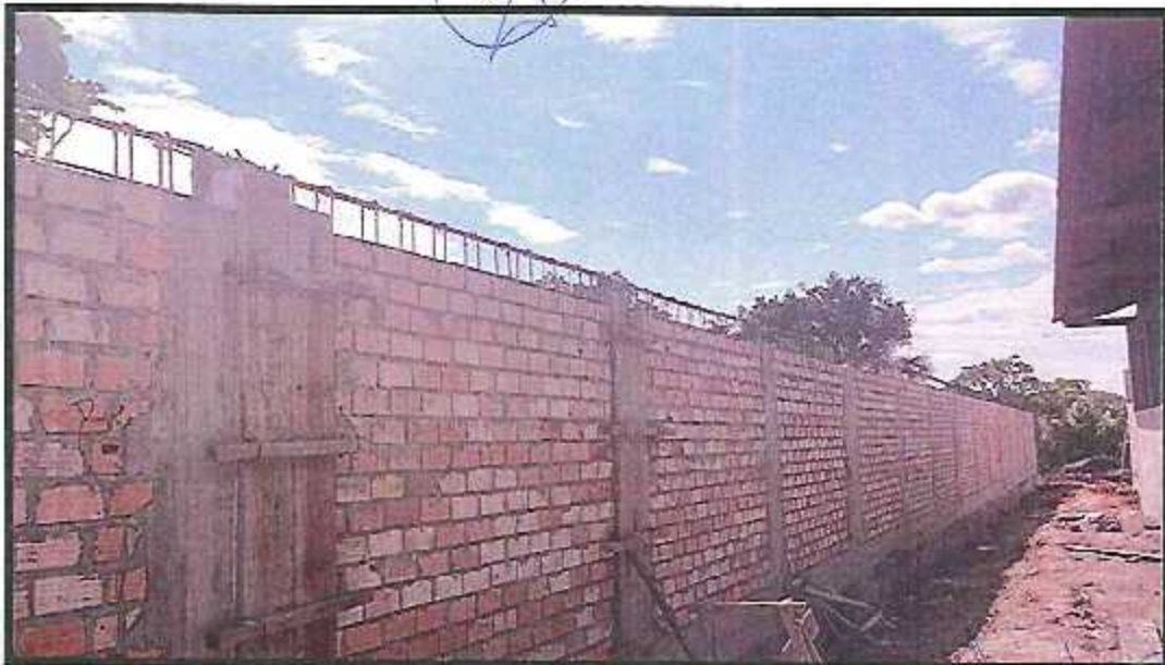
Viga de amarre en muro perimetrico
