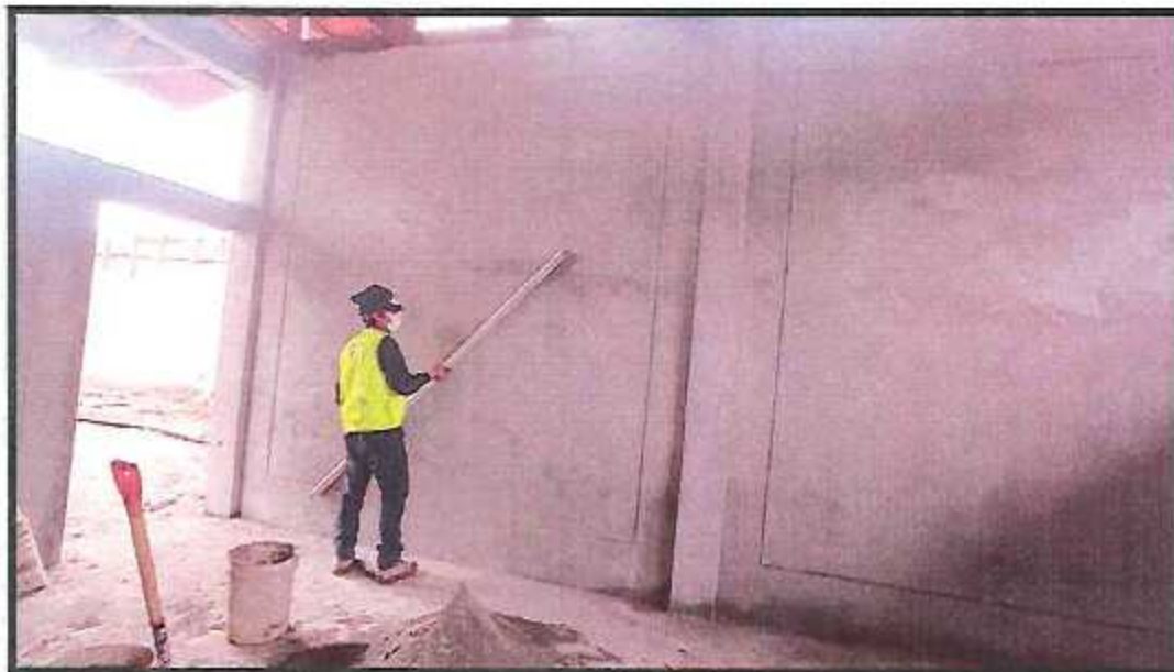
Tarrajeo en muro interior en módulos.
